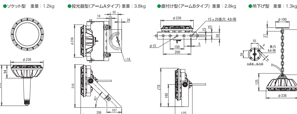
外形寸法図
