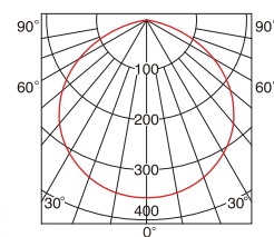
配光曲線 ※単位: cd/1000 ℓm
